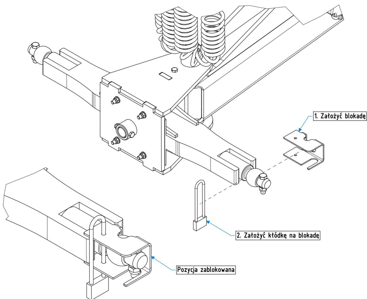
Rys. 89. Blokada dyszla
