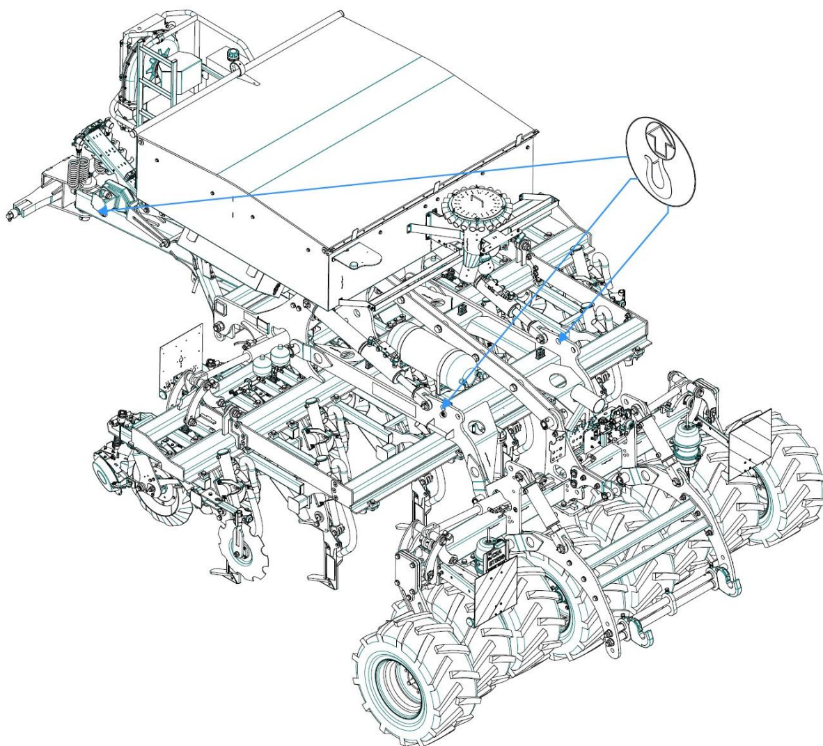
Rys. 91. Punkty unoszenia maszyny
