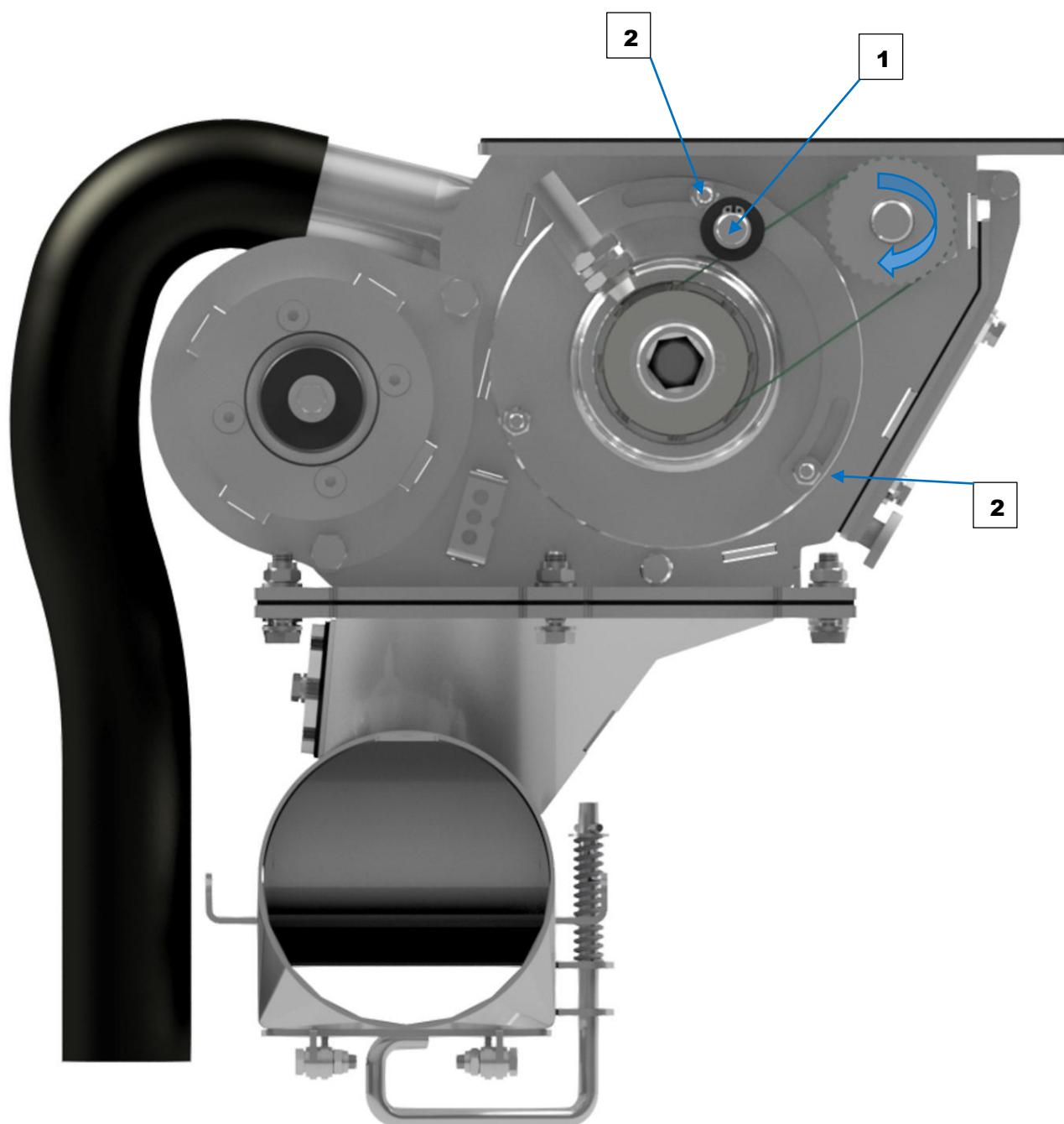
Rys. 60. Napinacz.
