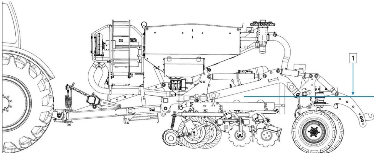
Rys. 79. Wypoziomowanie maszyny
