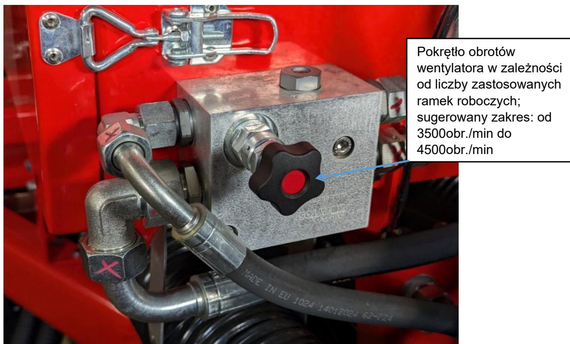
Rys. 42. Układ regulacji prędkości wentylatora oraz wentylatora lub WOM maszyny zaczepianej.
