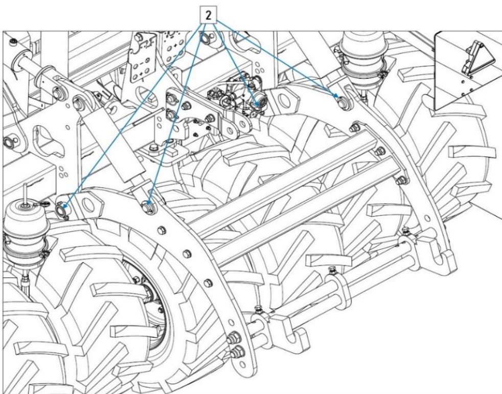
Rys. 80. Demontaż TUZ
