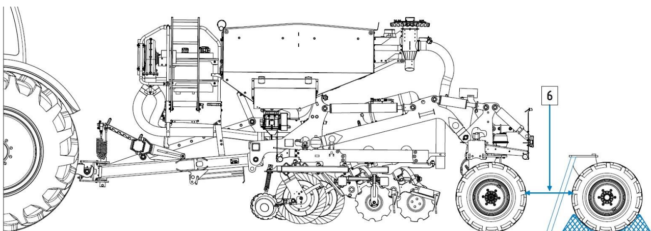
Rys. 84. Przejazd maszyny od zdemontowanego zespołu kołowego
