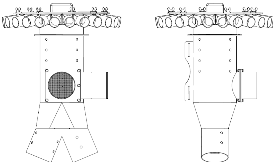
Rys. 65. Głowica rozdzielacza nasion
