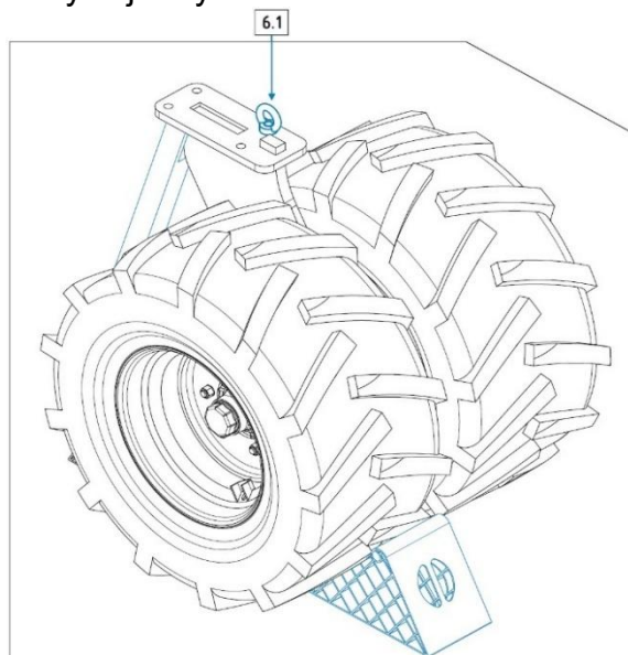
Rys. 85. Uniesienie zespołu kołowego za pomocą śruby/nakrętki z uchem
