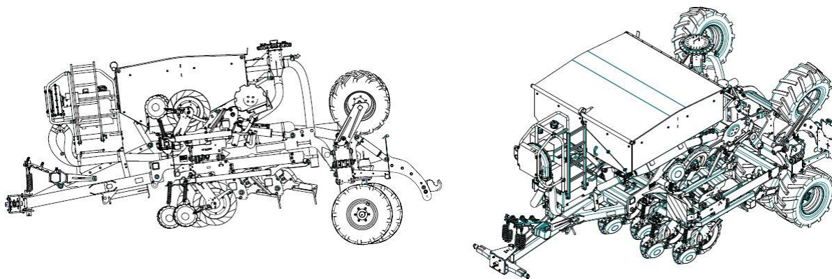
Rys. 71. Widok maszyny STK 400 w pozycji transportowej
