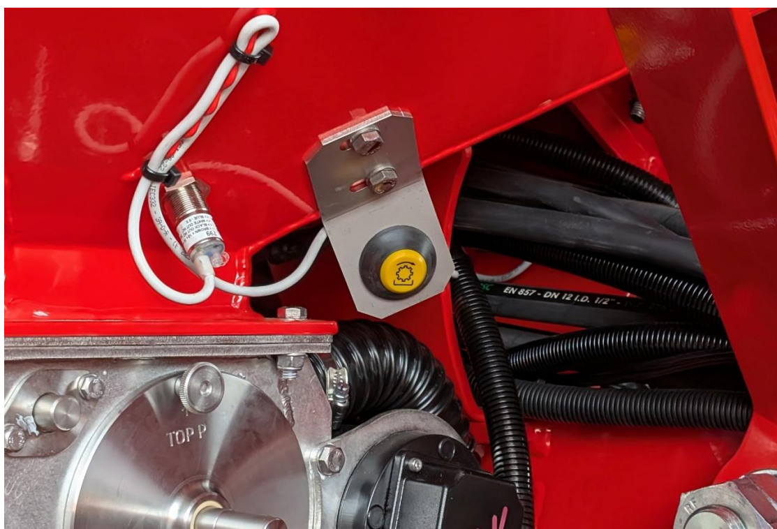
Rys. 64. Przycisk próby kręconej
