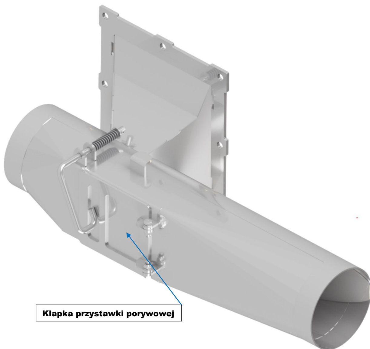
Rys. 61. Klapka przystawki porywowej.
