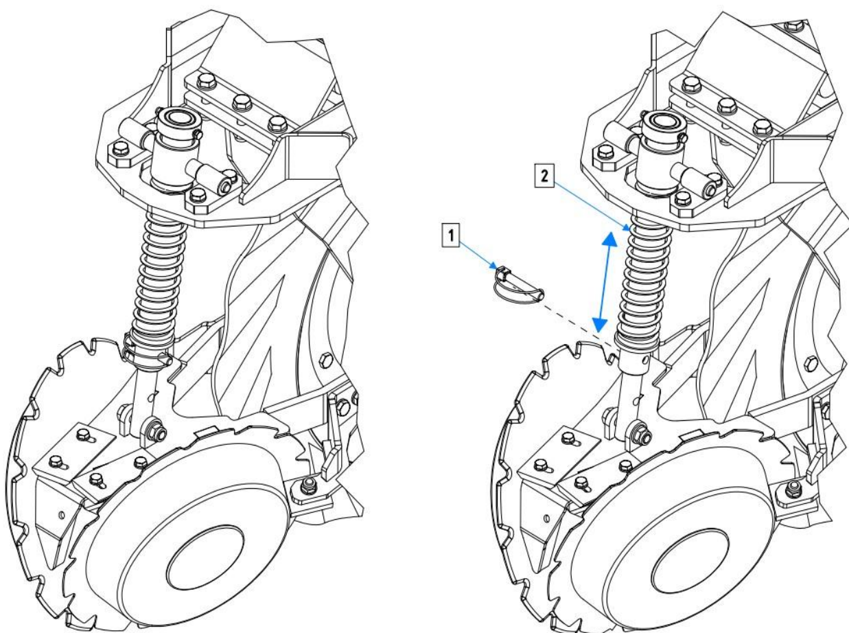
Rys. 75. Sposób regulacji docisku talerzy
