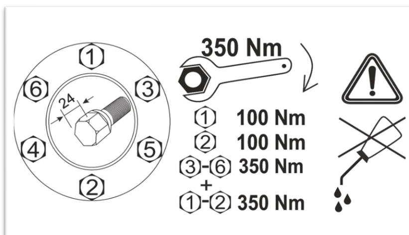
Rys. 88. Schemat dokręcania nakrętek kół STK
