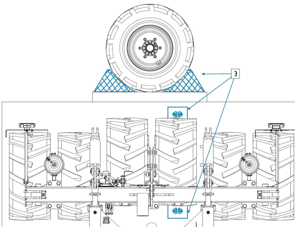
Rys. 81. Zabezpieczenie klinami
