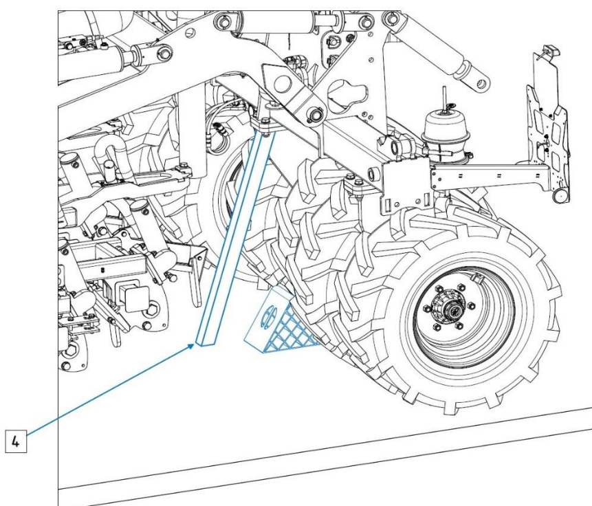
Rys. 82. Zabezpieczenie podporą
