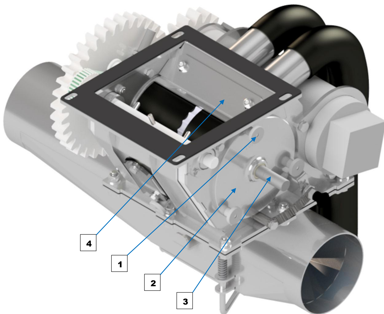
Rys. 54. Wymiana wałka wysiewającego.
