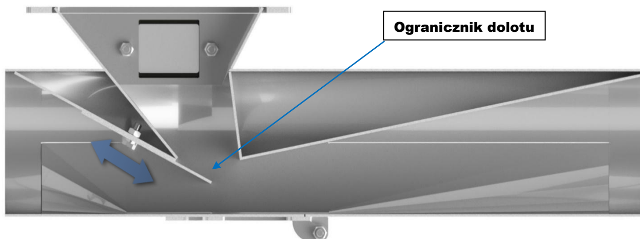
Rys. 62. Ogranicznik dolotu.
