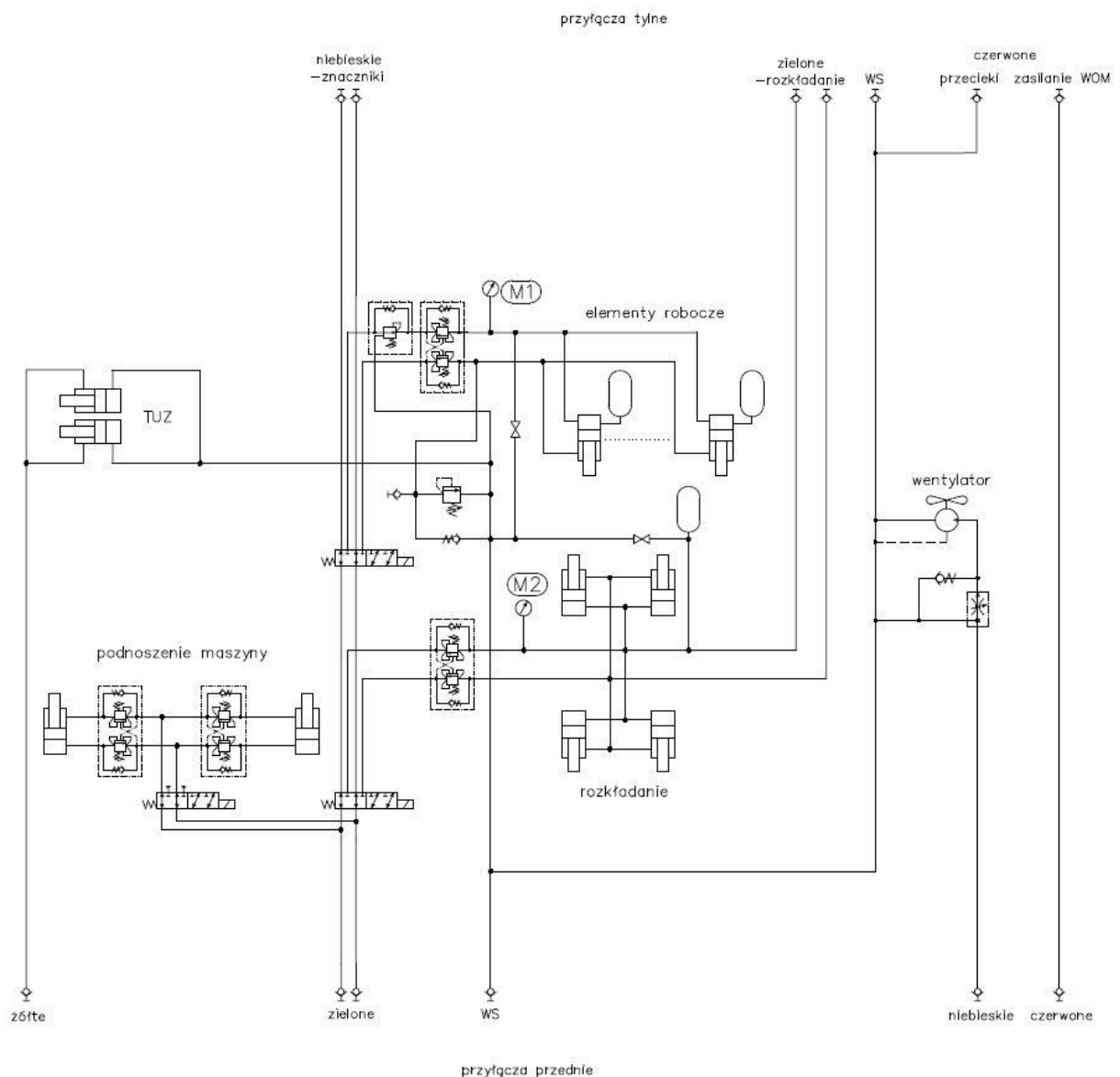
Rys. 37. Schemat układu hydraulicznego STK 400.
