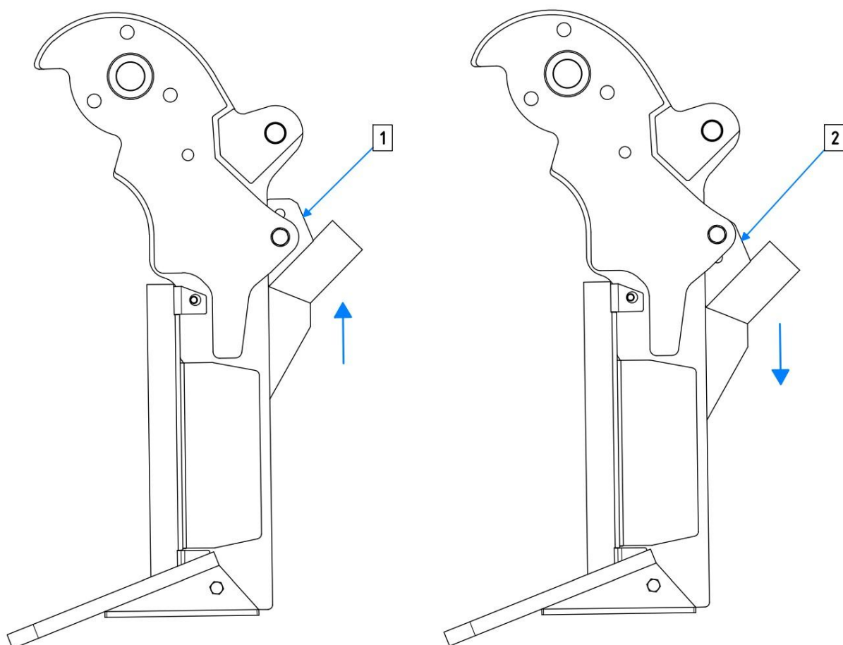
Rys. 74. Regulacja głębokości aplikowania nawozu
