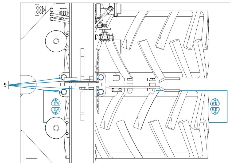
Rys. 83. Demontaż środkowego zespołu kołowego
