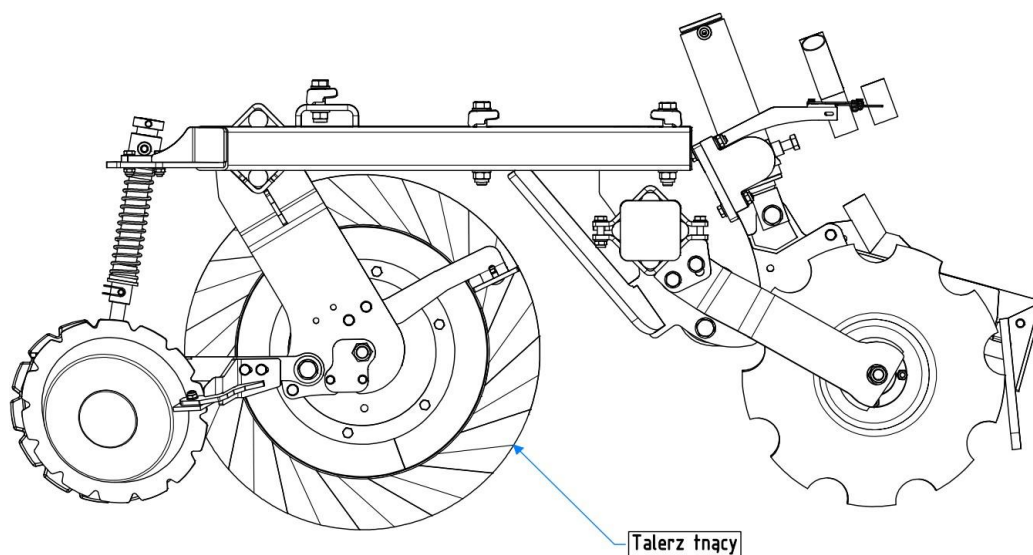
Rys. 76. Widok sekcji roboczej z boku
