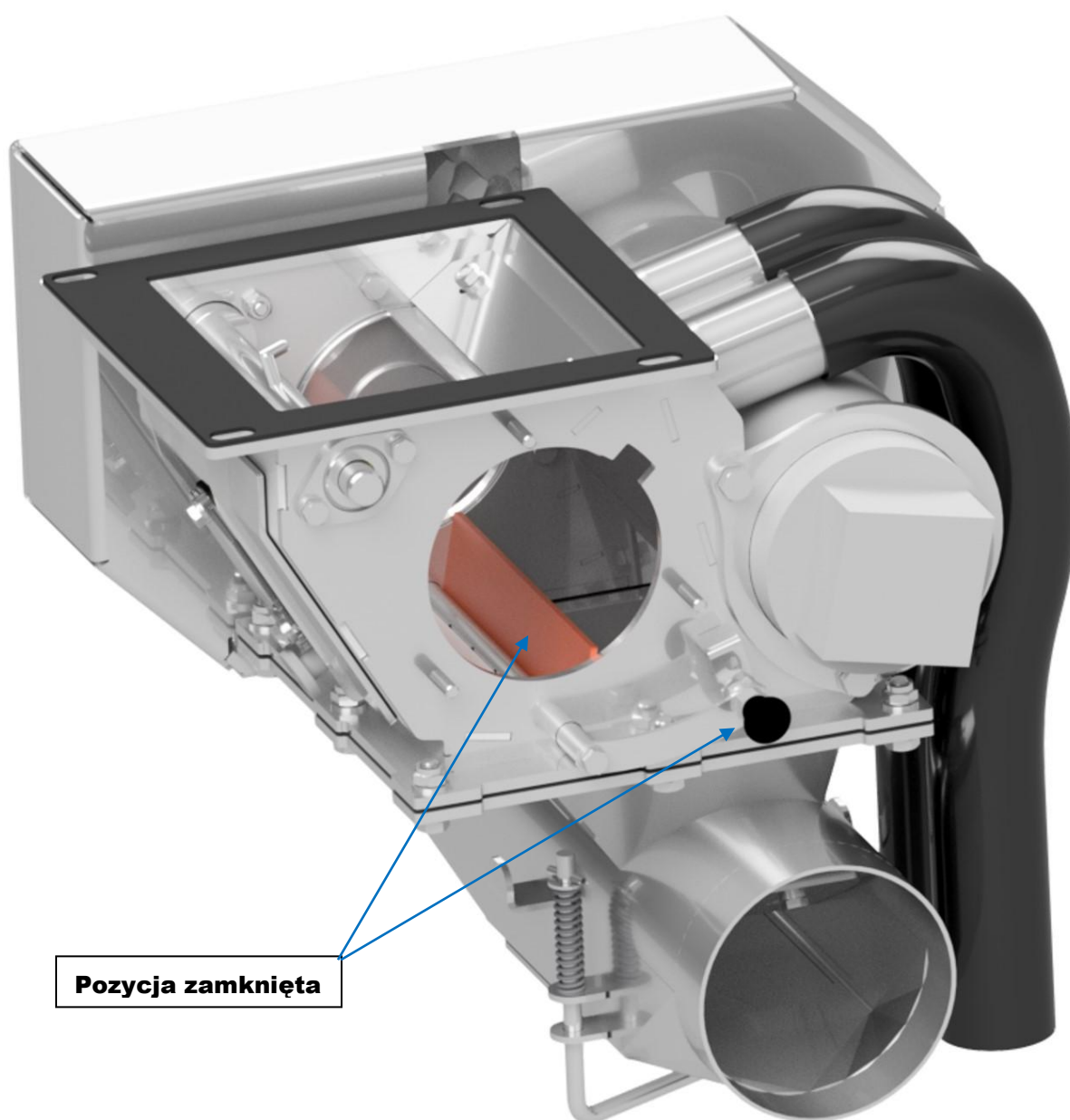
Rys. 66. Zgarniacz w pozycji zamkniętej
