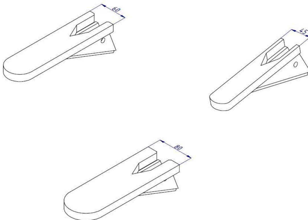
Rys.18. Rodzaje dostępnych dłut
