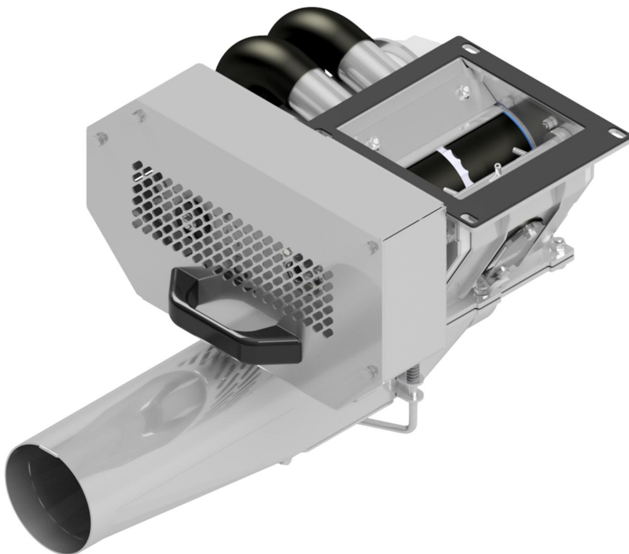
Rys. 57. Osłona kół zębatych
