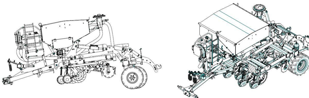
Rys. 70. Widok maszyny STK 300 w pozycji transportowej
