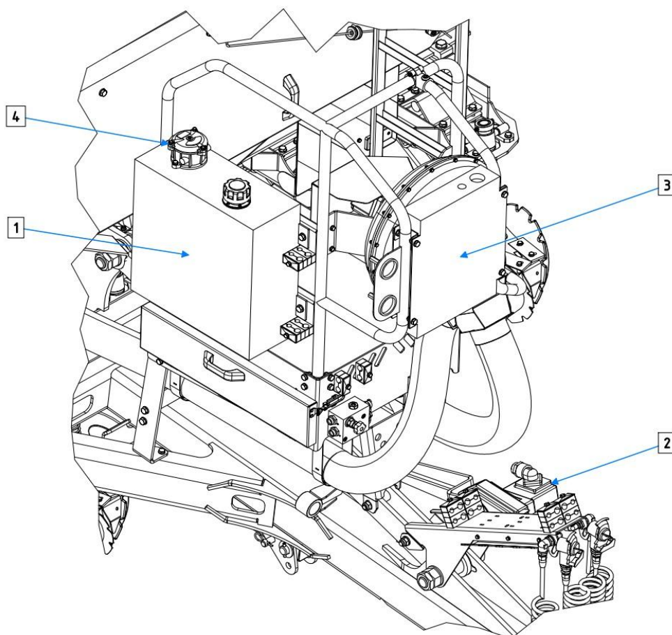
Rys. 52. Zewnętrzny układ hydrauliczny
