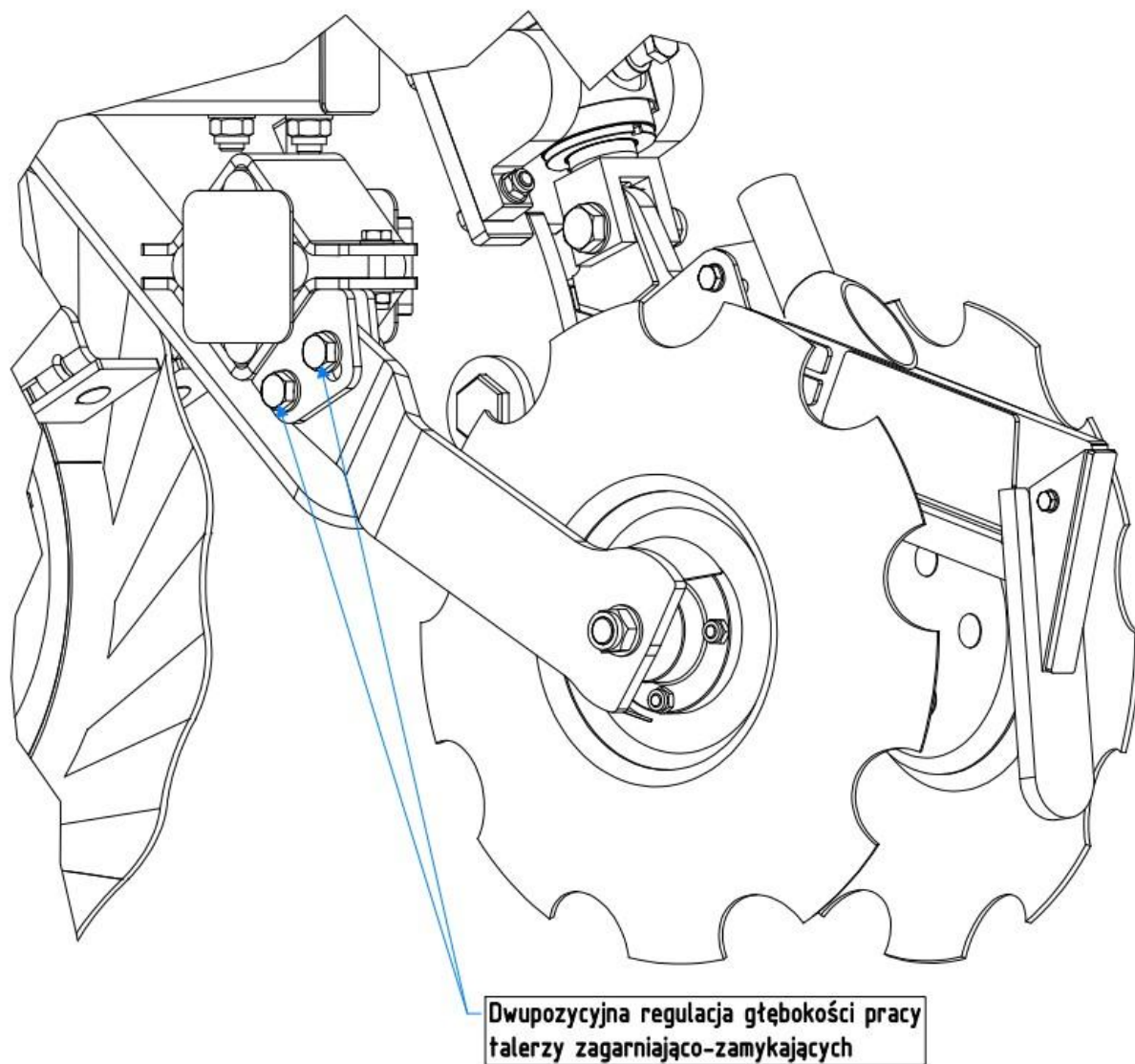
Rys. 77. Sposób regulacji głębokości pracy talerza zagarniająco zamykającego
