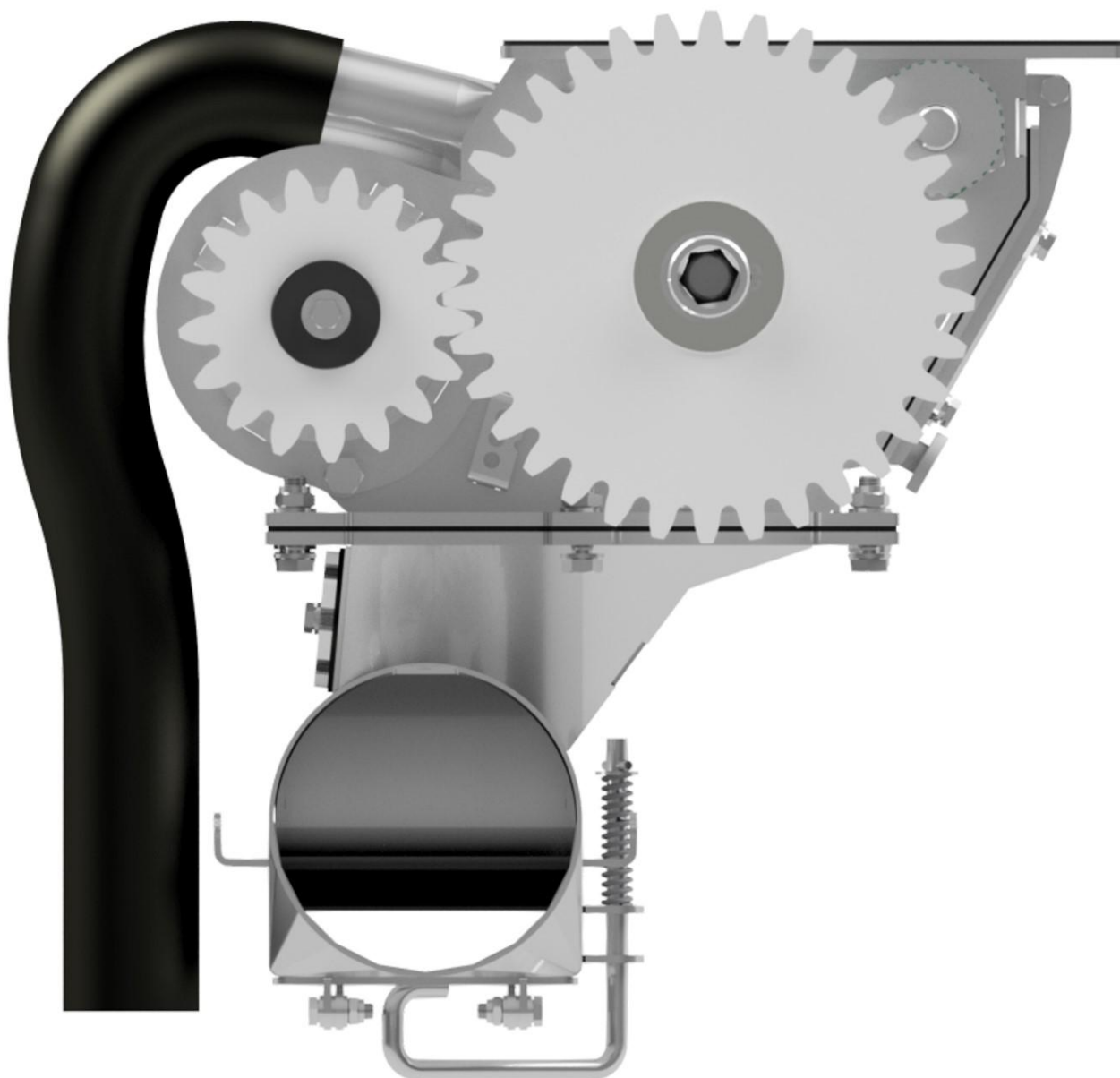
Rys. 56. Koła zębate aparatu wysiewającego.
