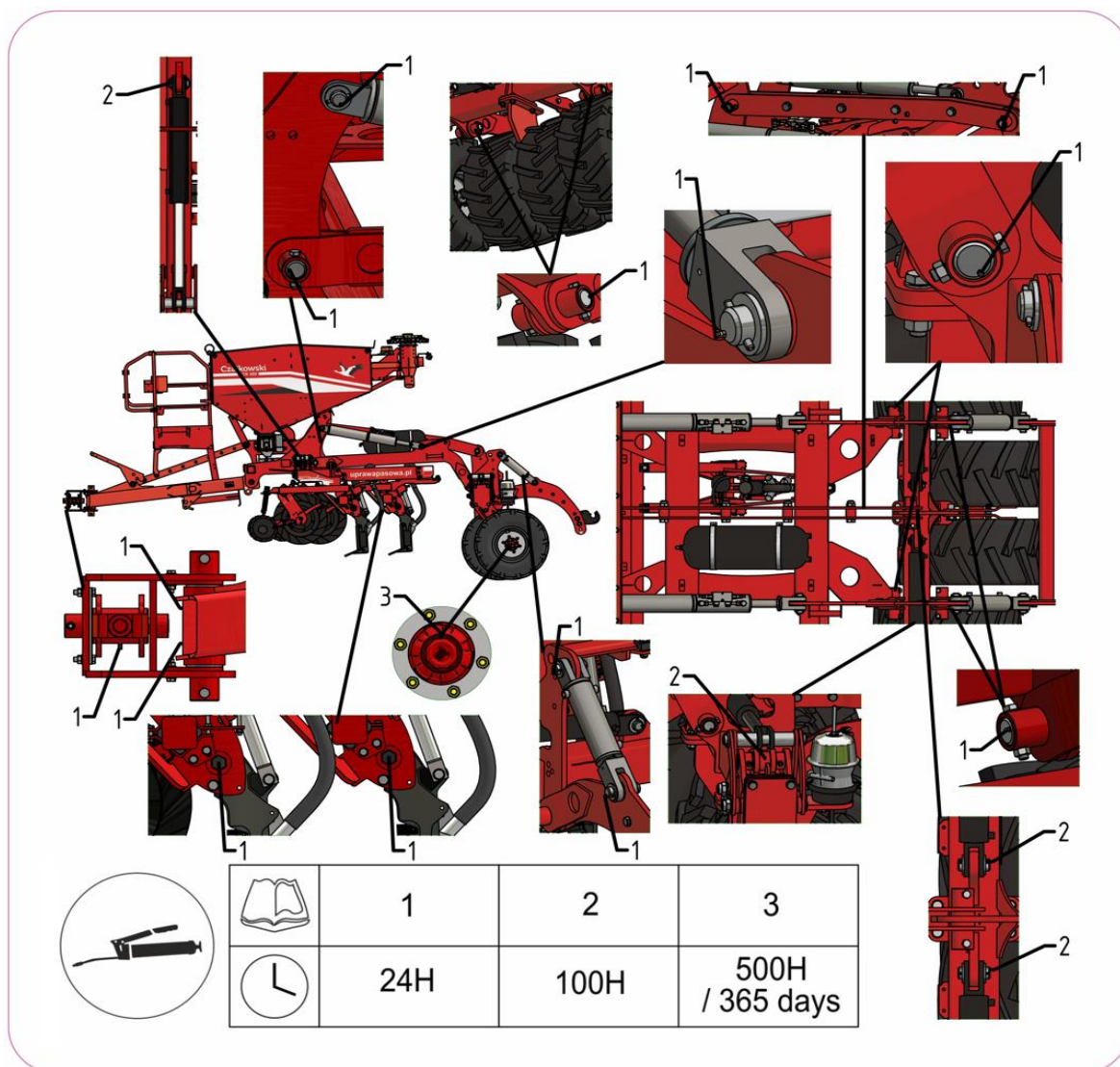
Rys. 68. Punkty smarne STK
