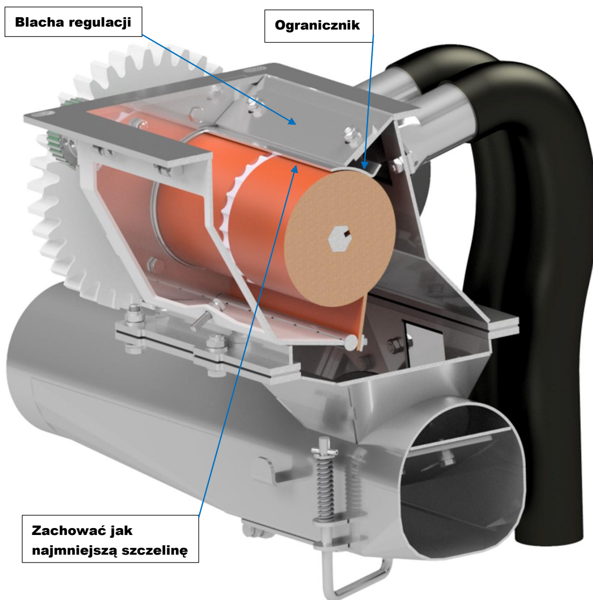
Rys. 59. Regulacja ogranicznika.
