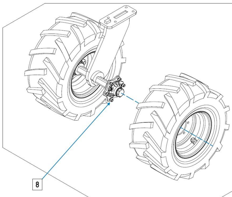
Rys. 87. Demontaż pojedynczego koła z zespołu kołowego
