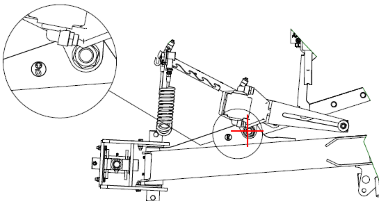
Rys. 92. Przedni punkt unoszenia maszyny
